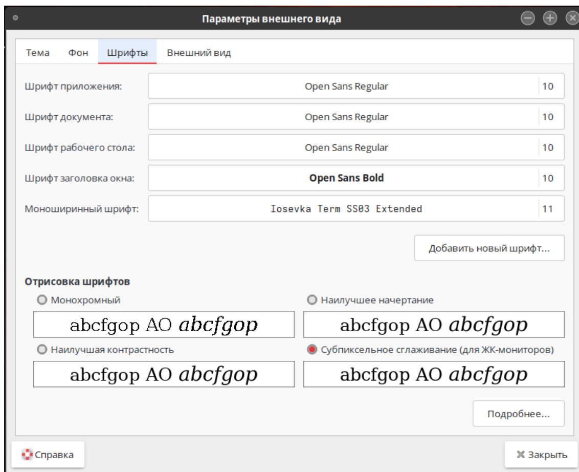
Рисунок 3.17 – Утилита настройки системных шрифтов
